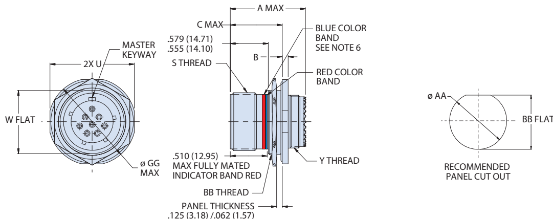
07 & 007 - JAM NUT MOUNT RECEPTACLE DIMENSIONS
